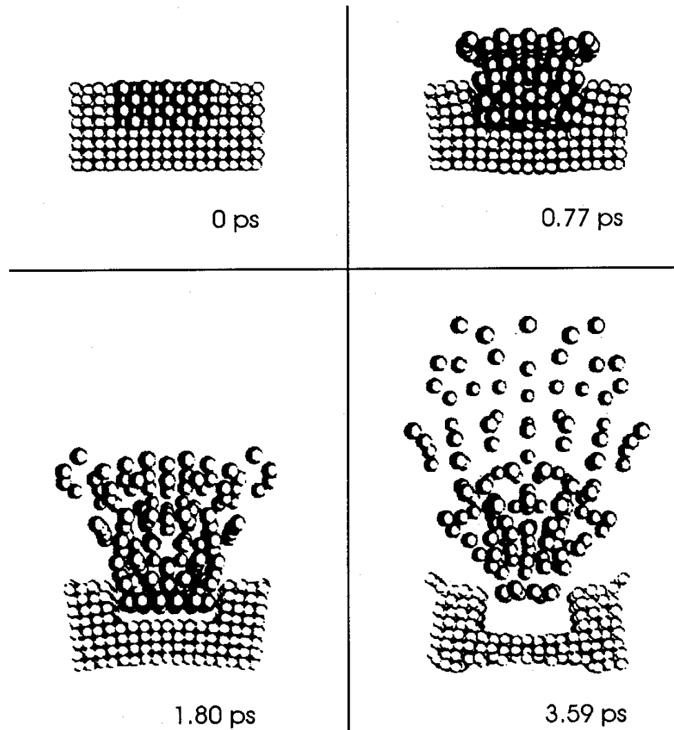
Abb II.4.2 Computer-Simulation der Photoablation von PMMA (Niemz[2])
